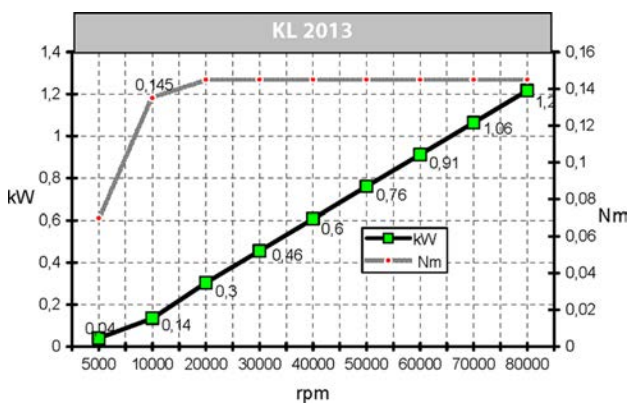
Диаграмма производительности
