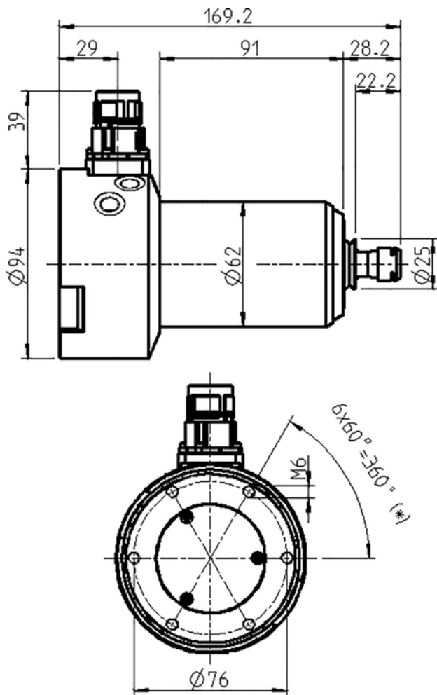
Размеры
