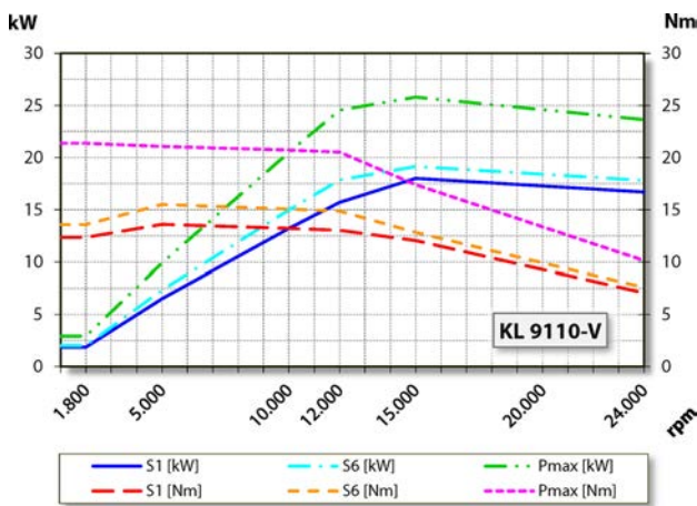
Wykres mocy
