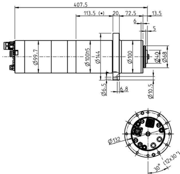
Abmessungen
