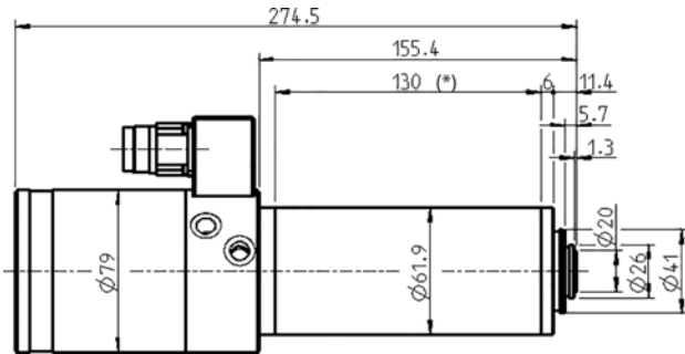
寸法図
