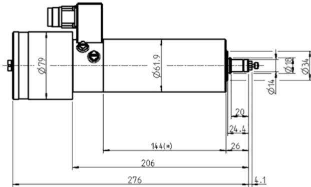
Dimensões
