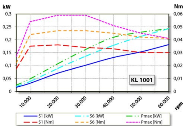
Diagrama de potência Não refrigerado
