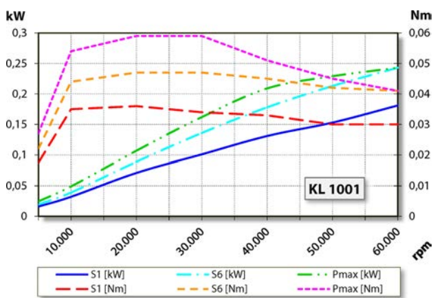
Diagramme de la courbe de puissance Non refroidi
