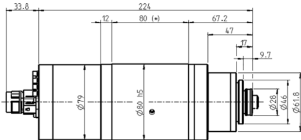
Abmessungen
