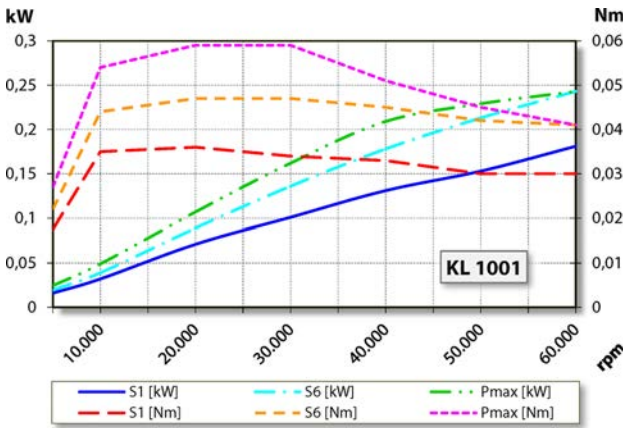
Güç diyagramı Soęutulmamıř
