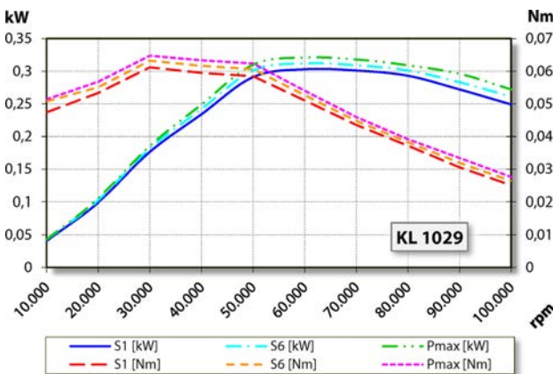
Диаграмма производительности Охлаждение крепежного кронштейна
