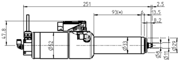
寸法図
