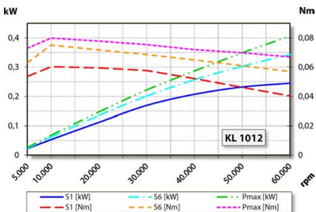
Diagram výkonu Nechlazen
