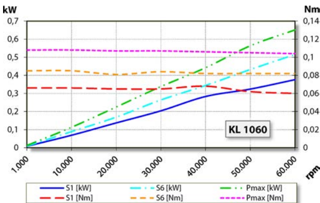
Diagrama de rendimiento Sin refrigerar
