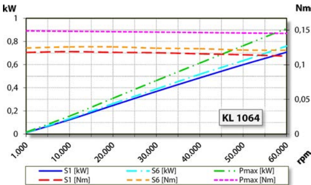
Diagrama de rendimiento Refrigeración de portahusillo
